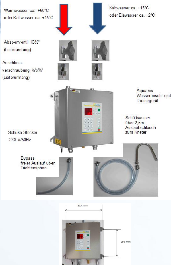
Anschluss-Schema
