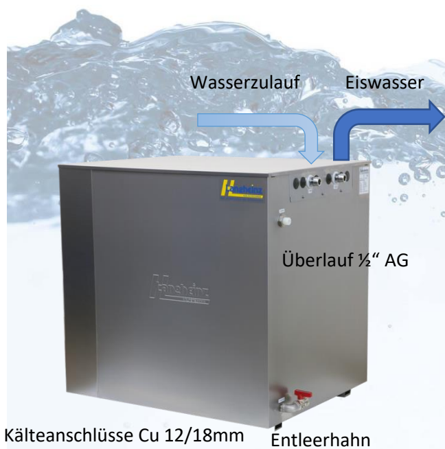
Ansicht hinten
